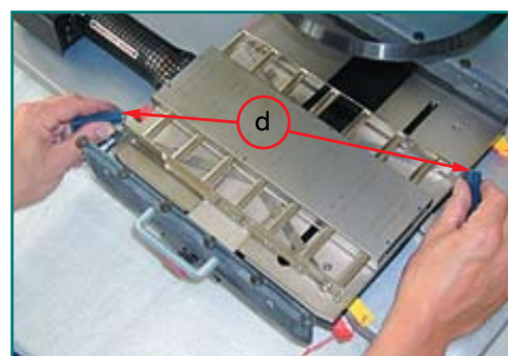
Рис. 4. Регулируемый нижний нагреватель
