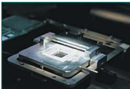
Рис. 8. Модуль трафаретной печати на компонент
